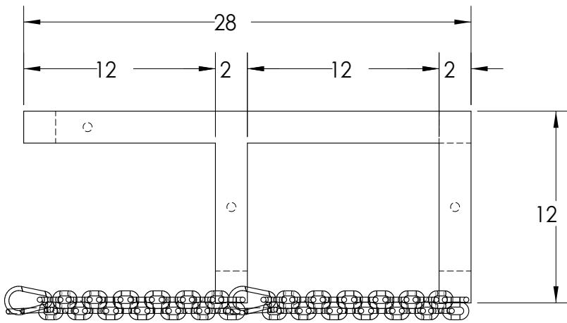
TOP
